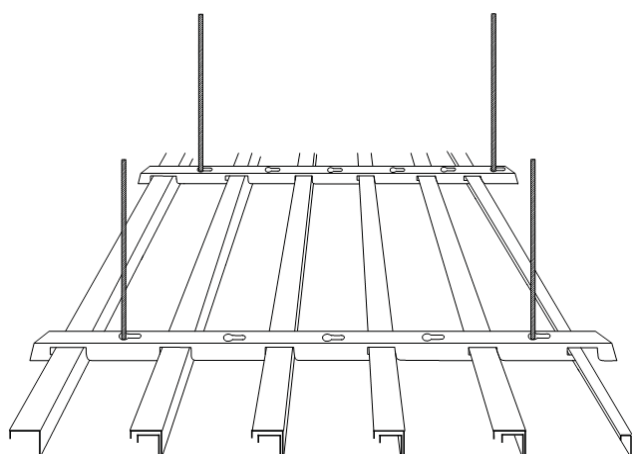
SOPORTE 200 ALUMINIO
